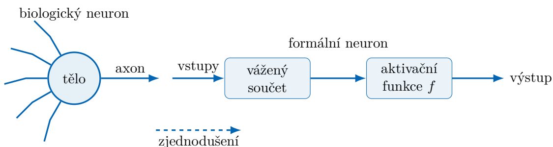
Figure 25: Biologická inspirace a její zjednodušení na formální neuron.
