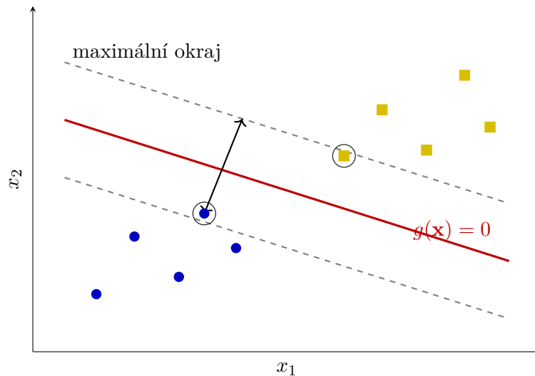
Figure 24: Oddělující přímka, maximální okraj a podpůrné vektory.
