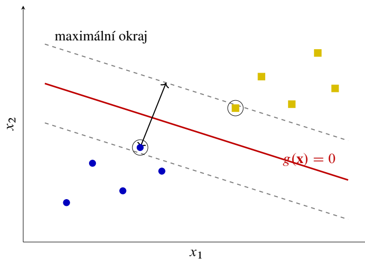
Obrázek 7.24: Oddělovací přímka, maximální okraj a podpůrné vektory.
