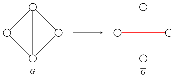
Obrázek 2.9: Doplňek grafu na čtyřech vrcholech.
