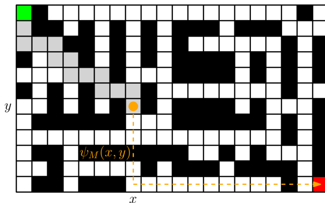
Obrázek 1.19: Příklad bludiště s manhattnskou heuristikou.
