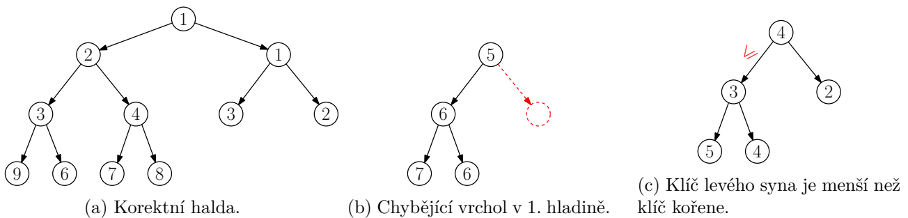
Obrázek 1.7: Příklady korektních a nekorektních hald.
