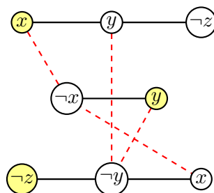
Figure 4: Ukázka nezávislé množiny příslušné splňujícím literálům pro formuli \psi .
