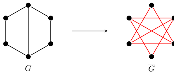
Figure 10: Doplněk prasátkového grafu.
