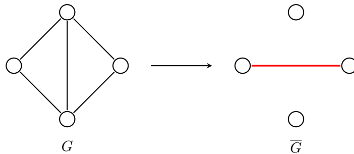
Figure 9: Doplněk grafu na čtyřech vrcholech.
