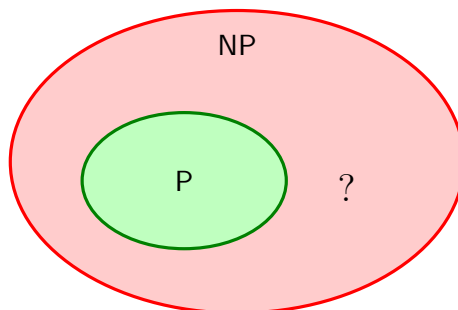
Figure 12: Schematická ilustrace vztahu P \subseteq NP ; zda je inkluze ostrá, nevíme.
