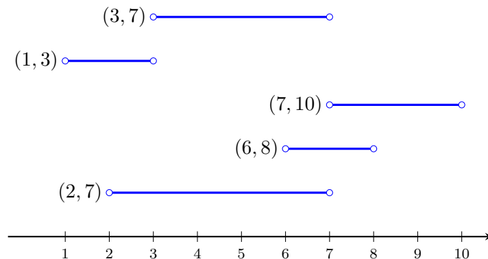
Figure 6: Příklad intervalového grafu pro intervaly (2, 7), (6, 8), (7, 10), (1, 3), (3, 7) .
