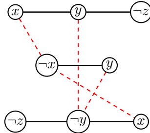
Figure 3: Ukázka sestrojeného grafu pro formuli \psi .
