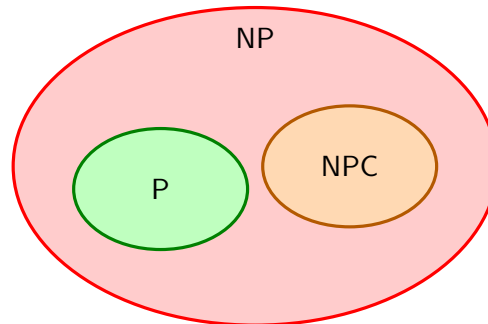
Figure 13: Obvyklé schematické znázornění vztahu P , NP a NPC za předpokladu P \neq NP .
