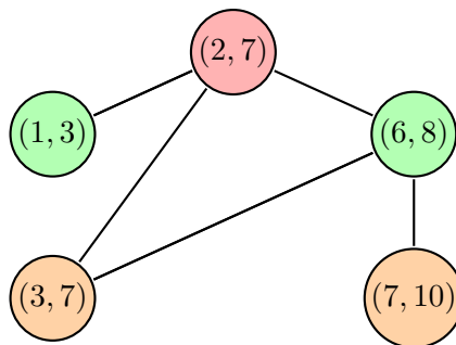
Figure 7: Obarvení intervalového grafu pro intervaly (2, 7), (6, 8), (7, 10), (1, 3), (3, 7) .
