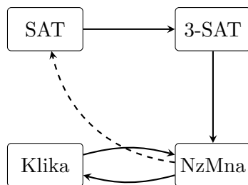
Figure 11: Shrnutí převodů mezi jednotlivými problémy.
