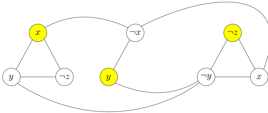
Obrázek 2.3: Ukázka nezávislé množiny příslušné splňujícím literálům pro formuli \varphi .
