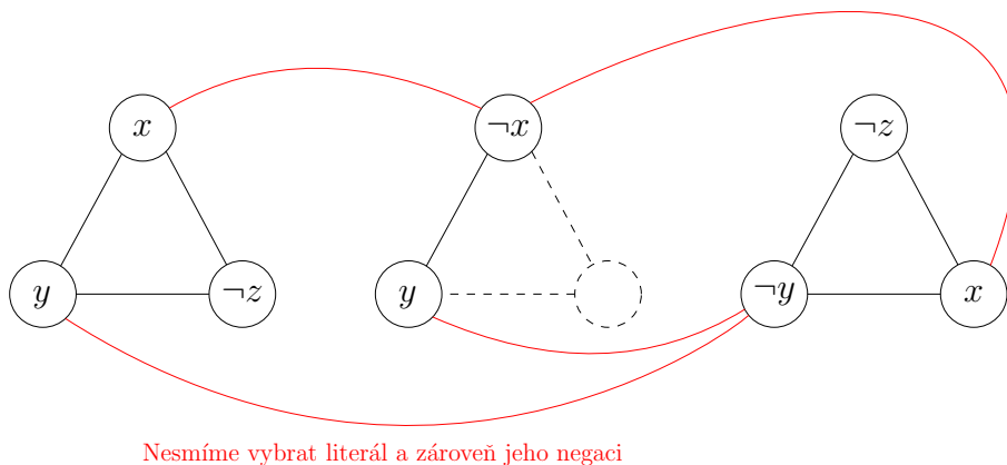
Obrázek 2.2: Ukázka sestrojeného grafu pro formuli \varphi .
