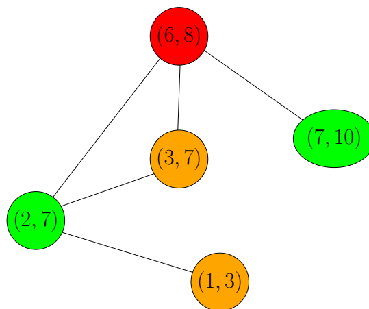
Obrázek 2.7: Obarvení intervalového grafu pro intervaly (2, 7) , (6, 8) , (7, 10) , (1, 3) , (3, 7) .
