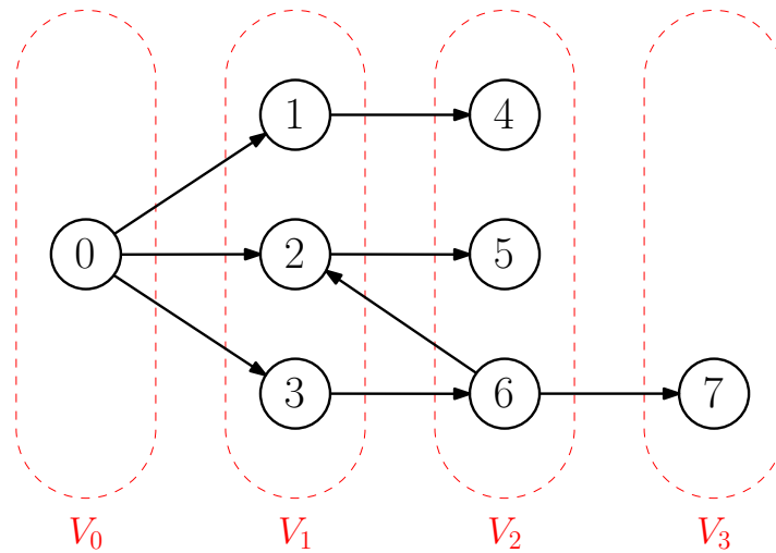
Obrázek 1.5: Vrcholy rozdělené do vrstev podle průběhu BFS.
