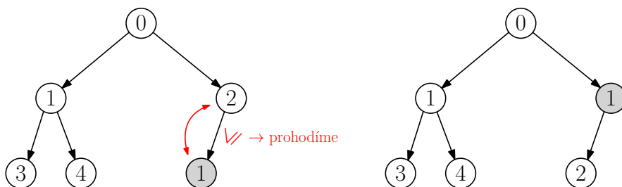
Obrázek 1.8: Vkládání nového vrcholu do haldy.
