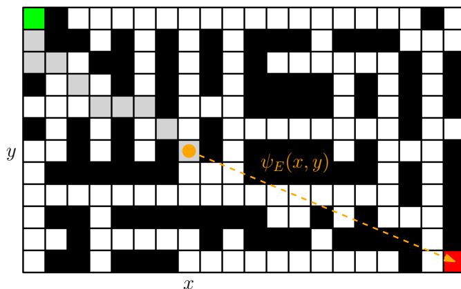
Obrázek 1.18: Příklad bludiště s eukleidovskou heuristikou.
