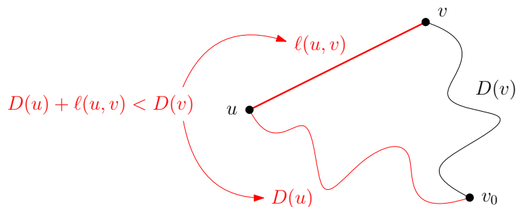
Obrázek 1.14: Situace při výběru vrcholu v , kdy D(v) neodpovídá délce nejkratší cesty.
