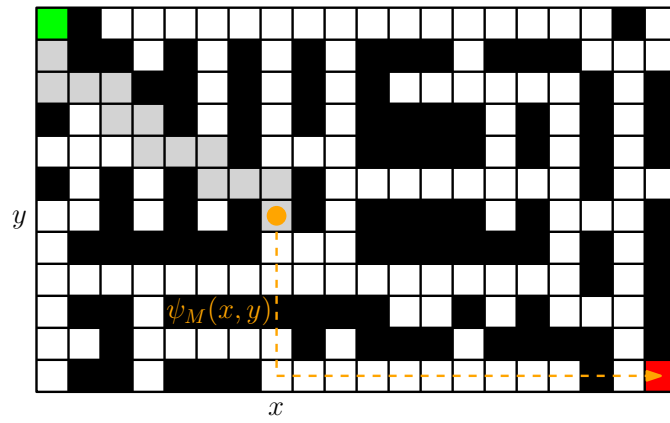
Obrázek 1.19: Příklad bludiště s manhattnskou heuristikou.
