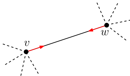
Obrázek 1.6: Znázornění situace v důkazu části (i) věty 1.3.1.
