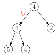
(c) Klíč levého syna je menší než klíč kořene.
