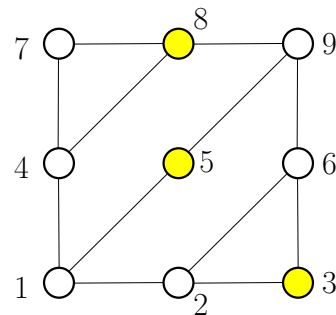
(b) Nezávislá množina vrcholů M_2 = \{3, 5, 8\} v G_2
