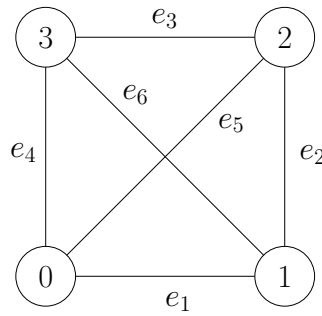
Obrázek 1.3: Úplný graf K_4 .
