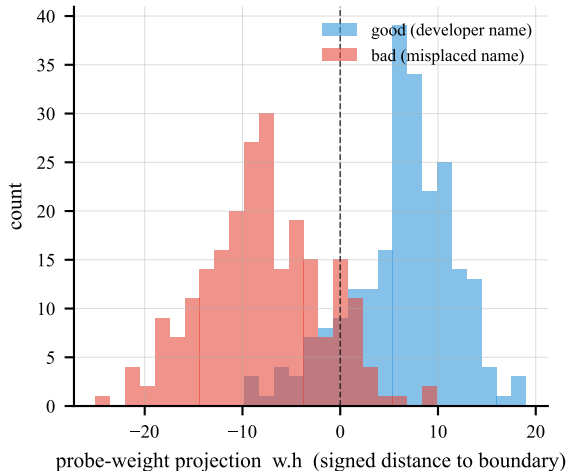
(b) Layer 28 separation (AUC=0.96)
