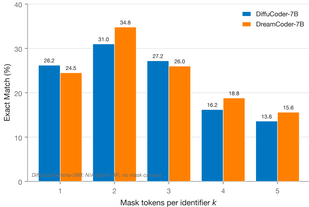
(a) EM vs. mask tokens per identifier
