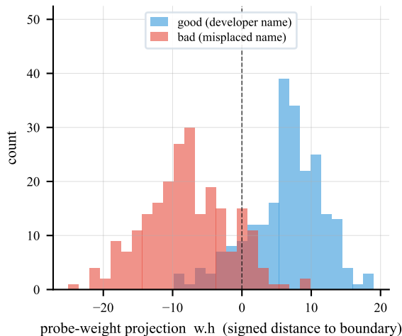
(b) Layer 28 separation (AUC=0.96)
