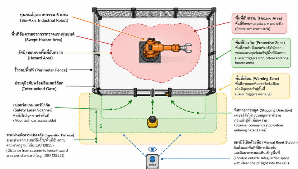
รูปที่ 7: Warning Zone และ Protective Zone ของเซลล์หุ่นยนต์
