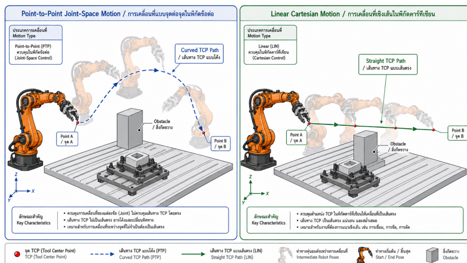
รูปที่ 2: เปรียบเทียบเส้นทาง PTP และ Linear
