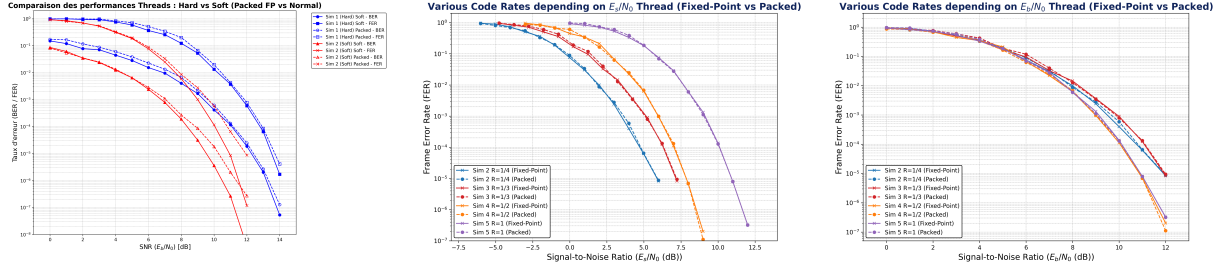
Fig. 8. – Résultats des simulations Thread Packed FP K = 32
