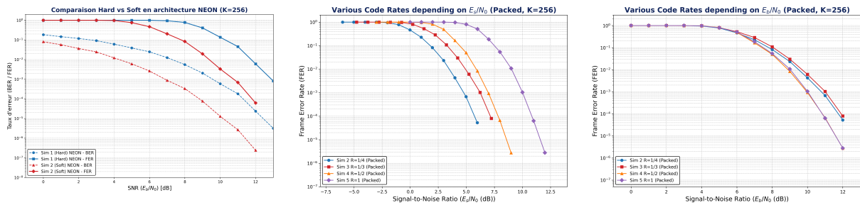
Fig. 2. – Résultats des simulations NEON pour K = 256
