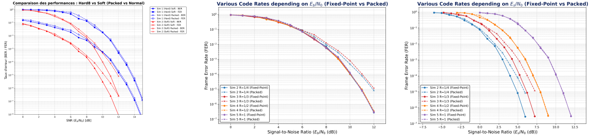
Fig. 5. – Résultats des simulations Packed Fixed-Point K = 32
