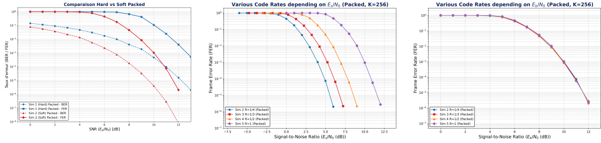
Fig. 4. – Résultats des simulations Packed Flottante K = 256
