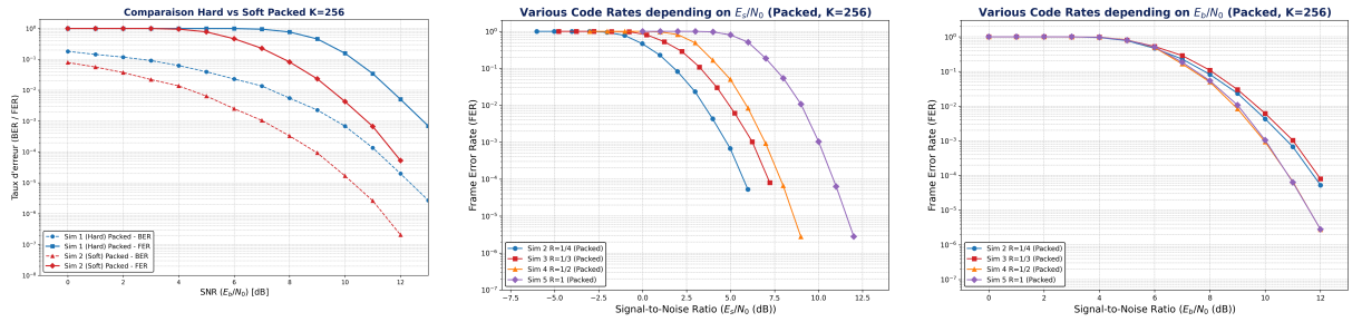
Fig. 6. – Résultats des simulations Packed Fixed-Point K = 256
