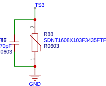
SHUNT温度
