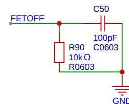
数字控制放电FET
