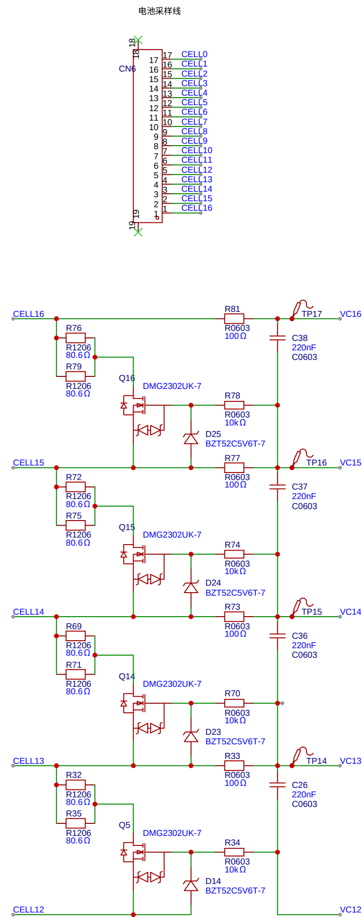
电池采样线
