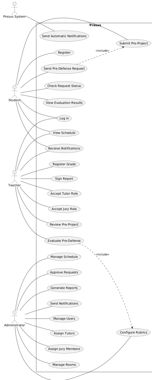
Fig. 8. Diagrama de casos de uso: actores y relaciones include/extend principales.
