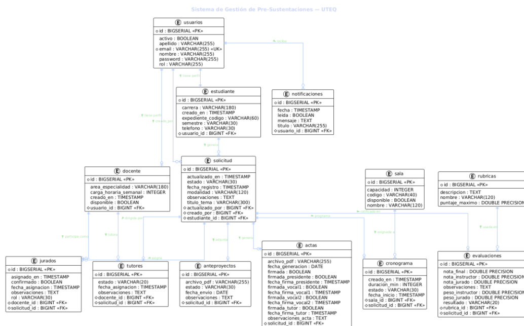
Fig. 7. Diagrama de entidad-relación del sistema de gestión de pre-sustentaciones.
