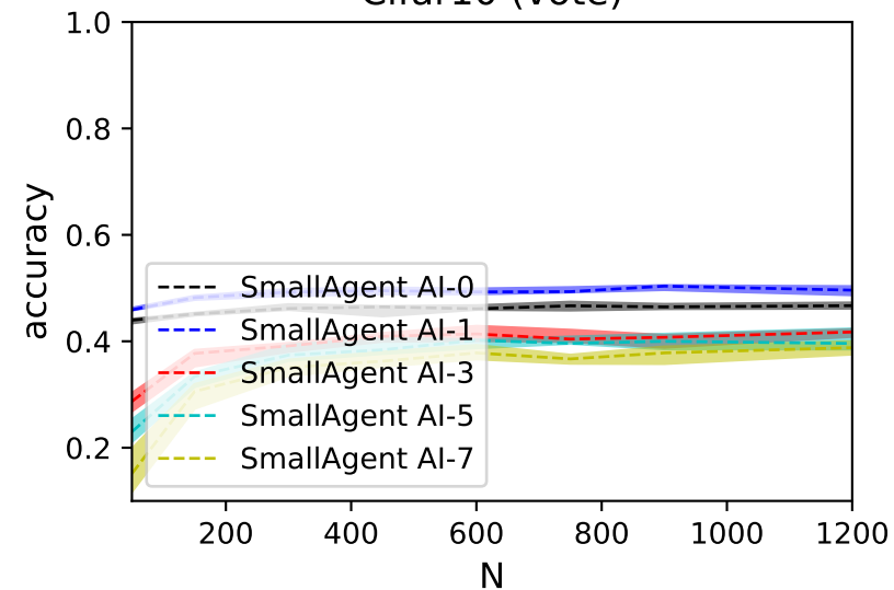
Cifar10 (vote)
