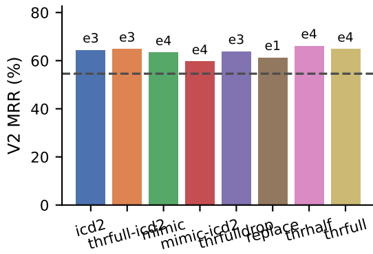
V2 MRR
