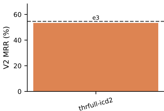
V2 MRR
