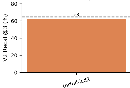
V2 Recall@3
