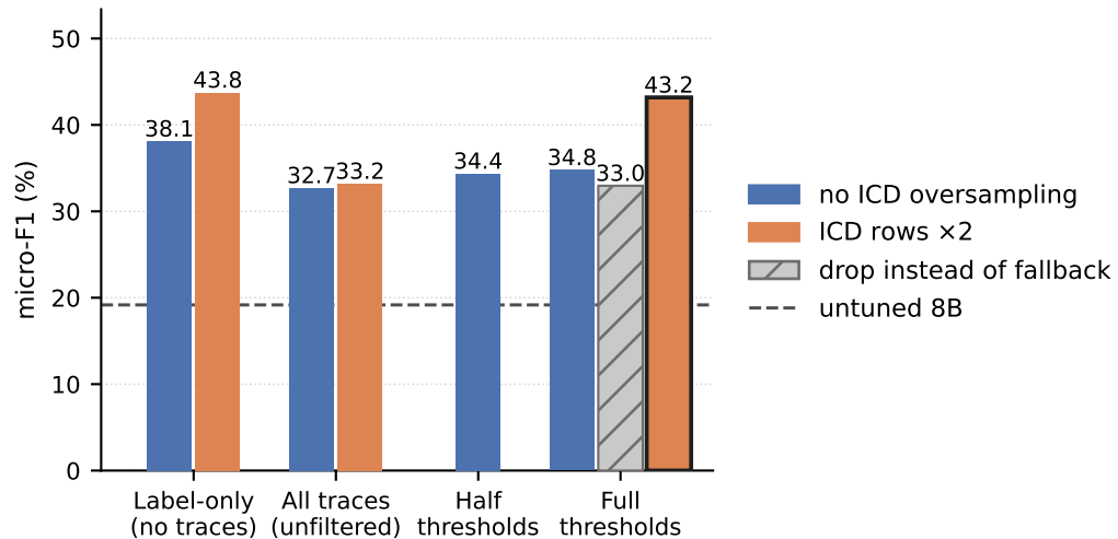
ICD codes: micro-F1
