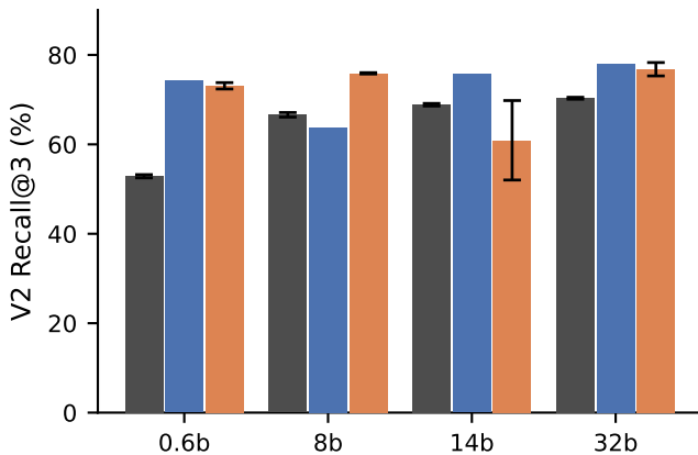
V2 Recall@3
