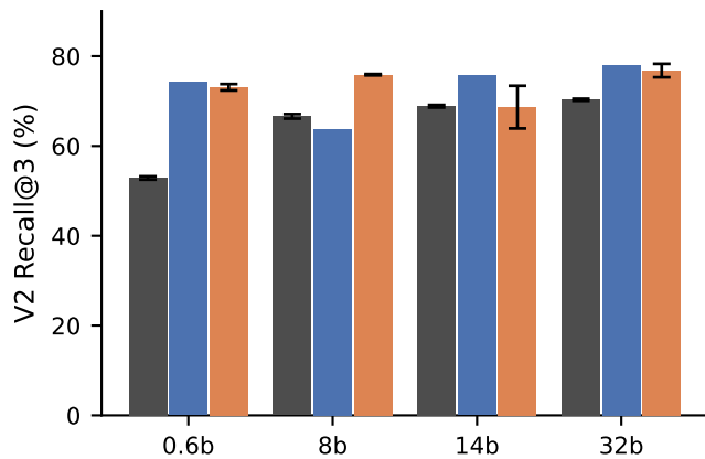
V2 Recall@3
