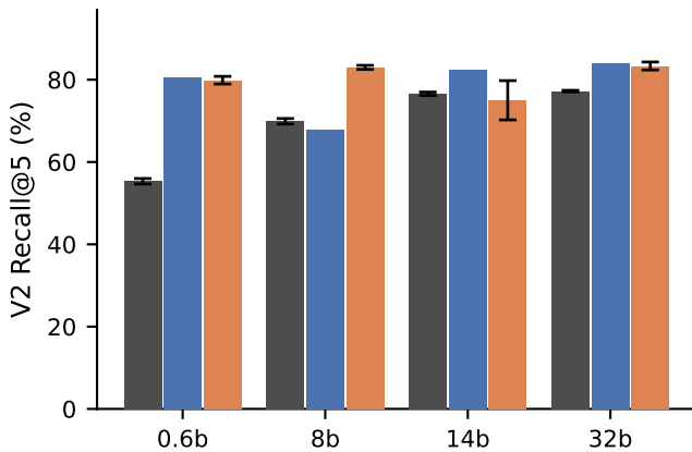
V2 Recall@5
