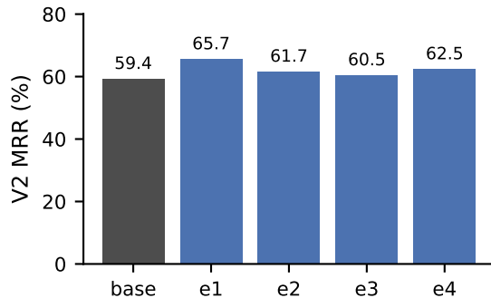
V2 MRR
