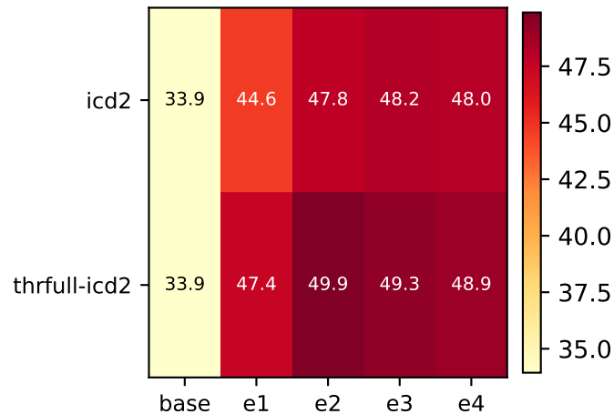
V2 MRR
