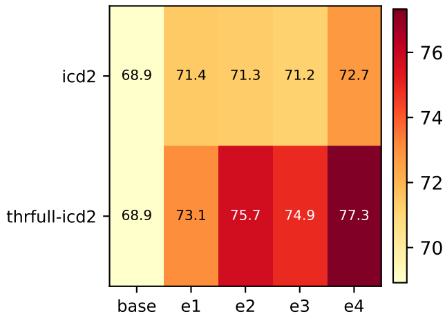
V2 Recall@3
