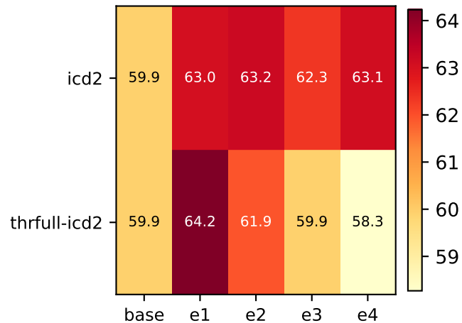
V2 MRR
