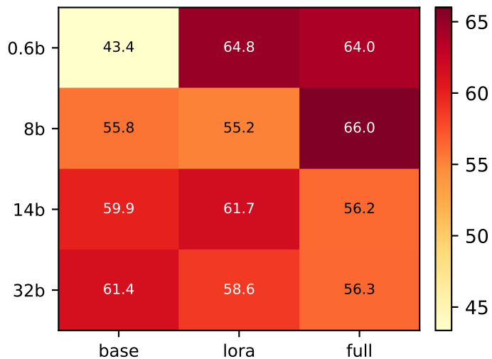
V2 MRR
