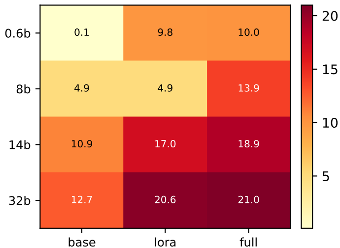
V2 Recall@3
