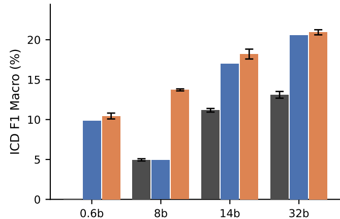
ICD F1 Macro
