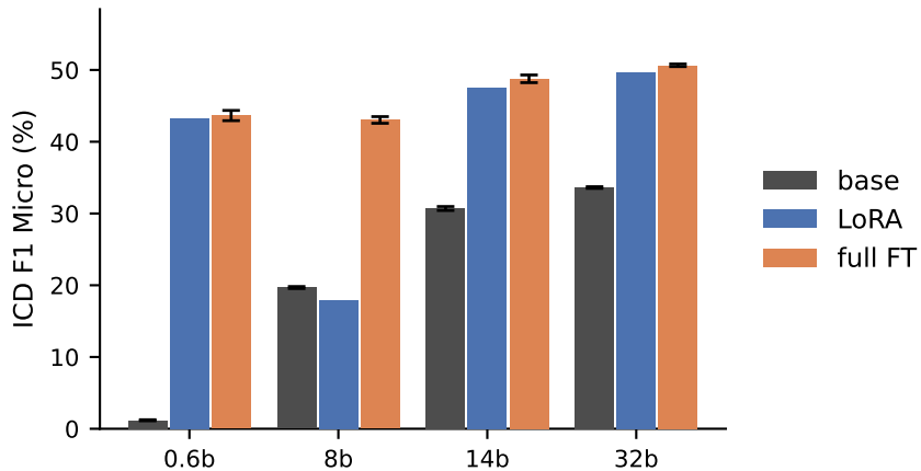
ICD F1 Micro
