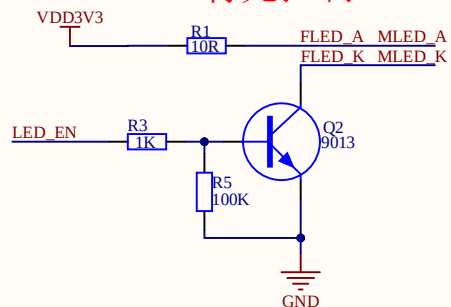
TFT 背光控制
