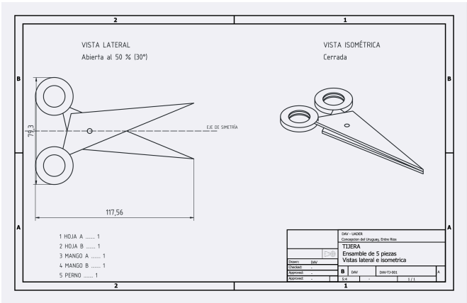
Plano de la tijera: vista lateral abierta al 50 % y vista isométrica cerrada
