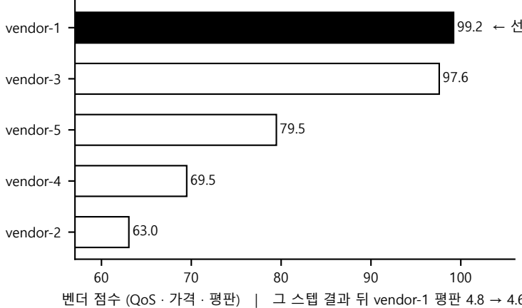
스텝 0 · URLLC 벤더 점수 (score_offerings) — vendor-1 선택 점수 1위 벤더에서 조달
