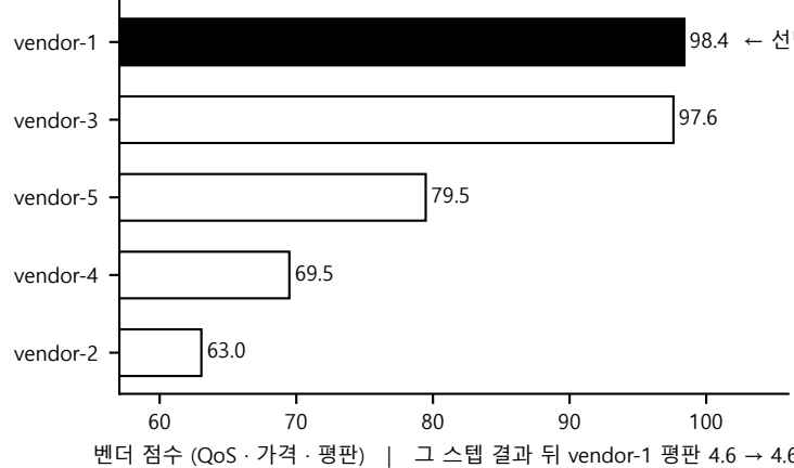
스텝 4 · URLLC 벤더 점수 (score_offerings) — vendor-1 선택 같은 벤더가 계속 1위
