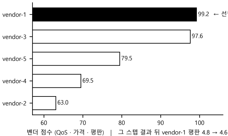
스텝 3 · URLLC 벤더 점수 (score_offerings) — vendor-1 선택 점수 1위 벤더에서 조달
