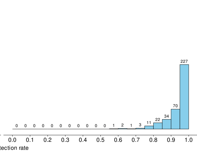
EpicV2
