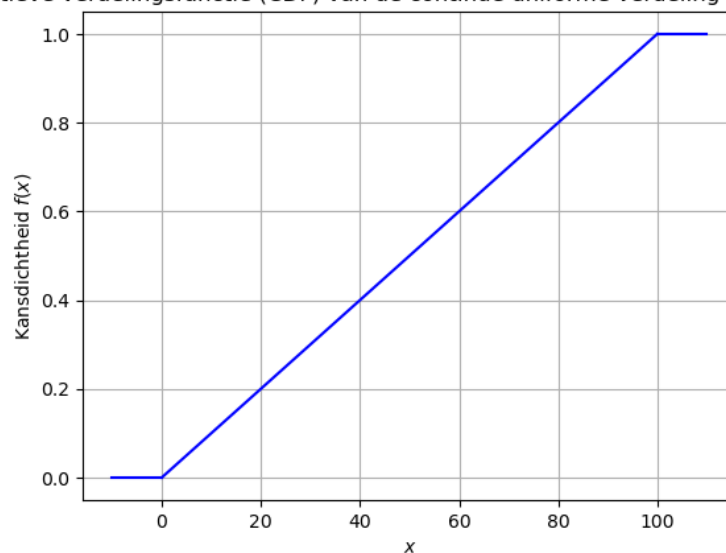
Cumulatieve verdelingsfunctie (CDF) van de continue uniforme verdeling tussen 0 en 100
