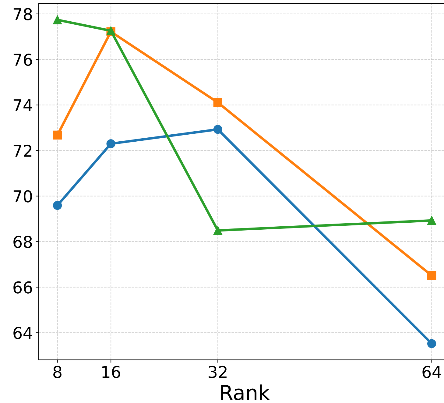
Pass@5 (%)
