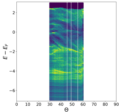
(d) DZVP, d = 2.25 Å
