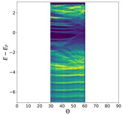
(d) d = 2.70 \text{ \AA}
