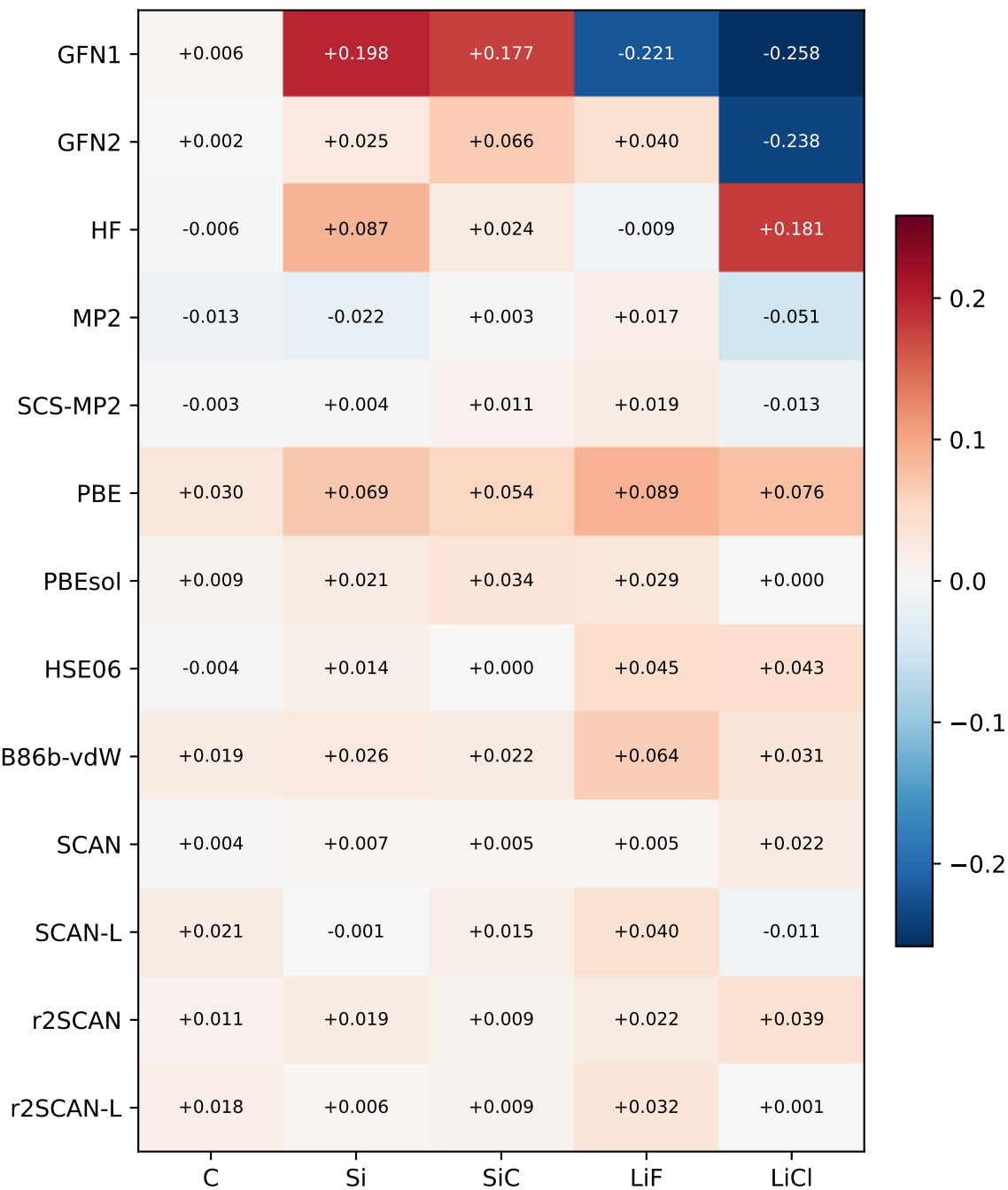
Lattice-constant error (Å)
