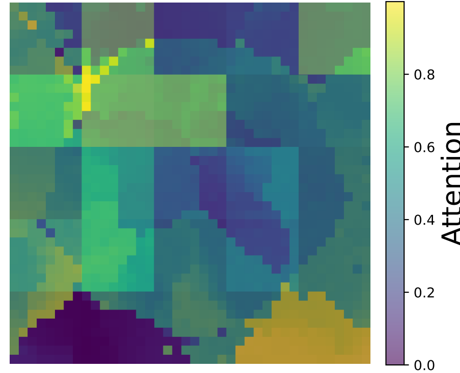
Layer 2 (Image)
