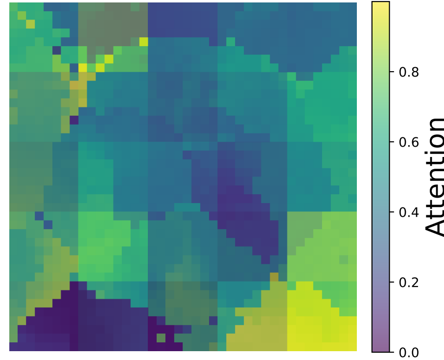
Layer 1 (Image)
