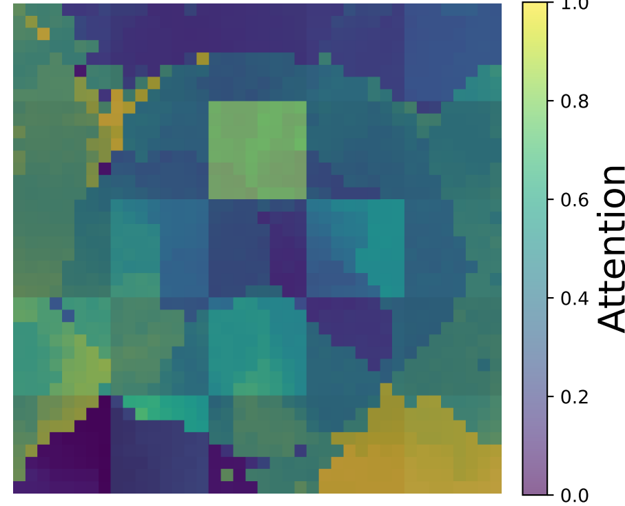
Layer 2 (Image)
