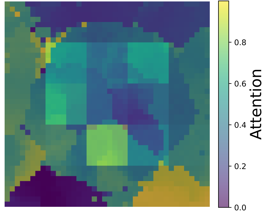
Layer 3 (Image)
