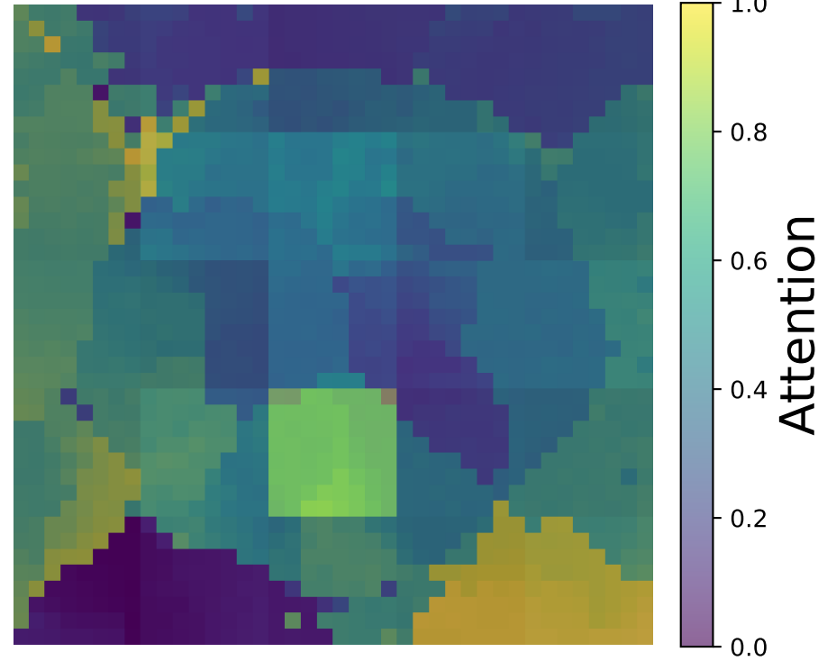
Layer 4 (Image)
