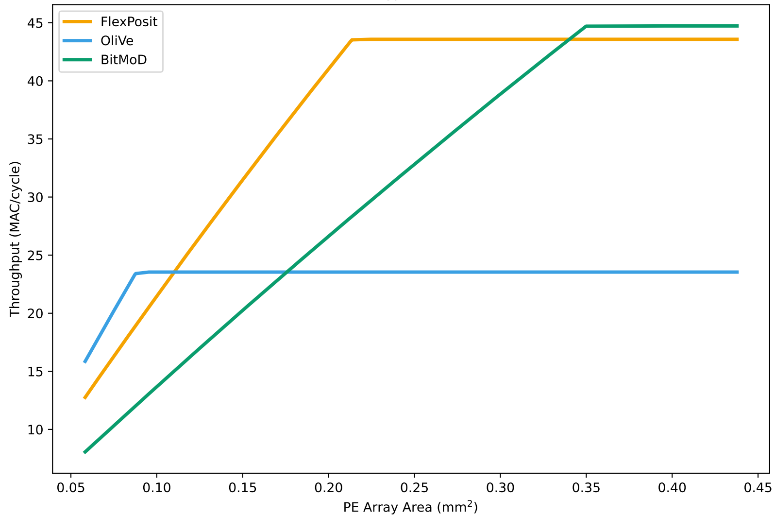
gpt2-xl
