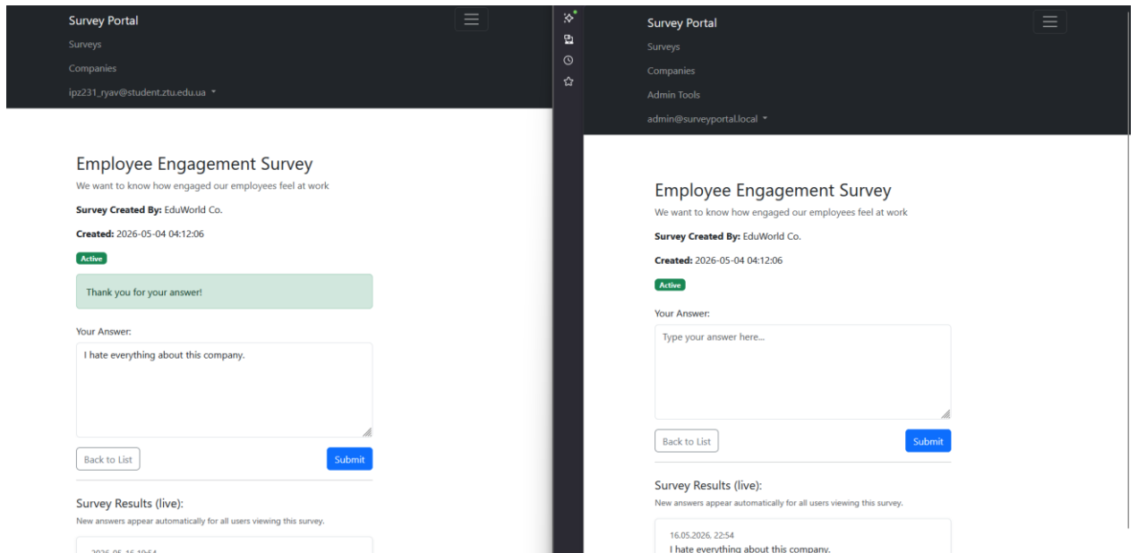
Рис. 3. Два вікна браузера з однаковою сторінкою опитування: після відправки відповіді у першому вікні нова відповідь з'являється у другому без перезавантаження сторінки.
