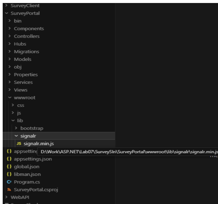
Рис. 1. Структура проекту SurveyPortal з папкою Hubs та підключеним клієнтом SignalR у wwwroot/lib/signalr.
