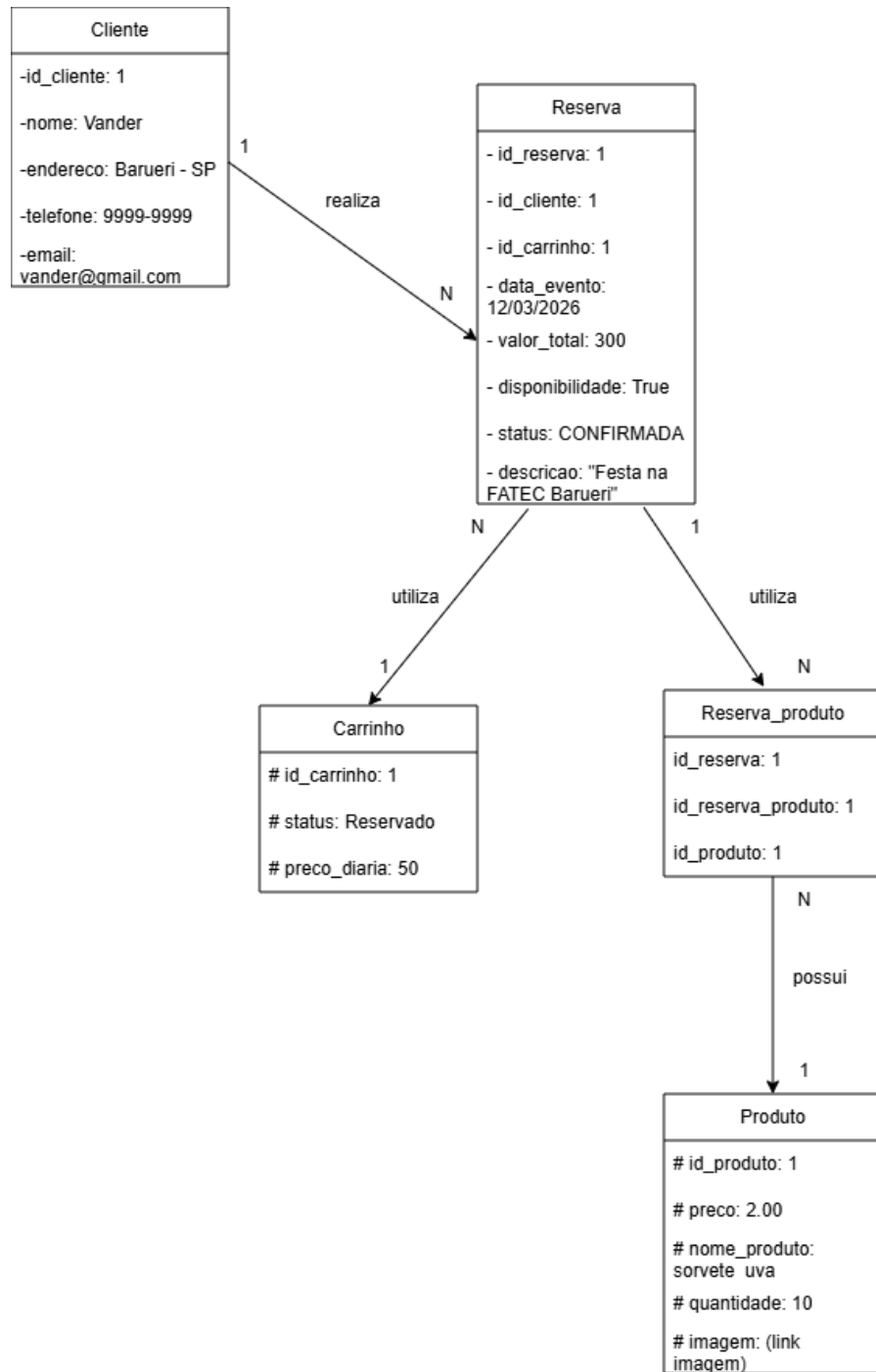
Imagem 02 – Diagrama de objetos
