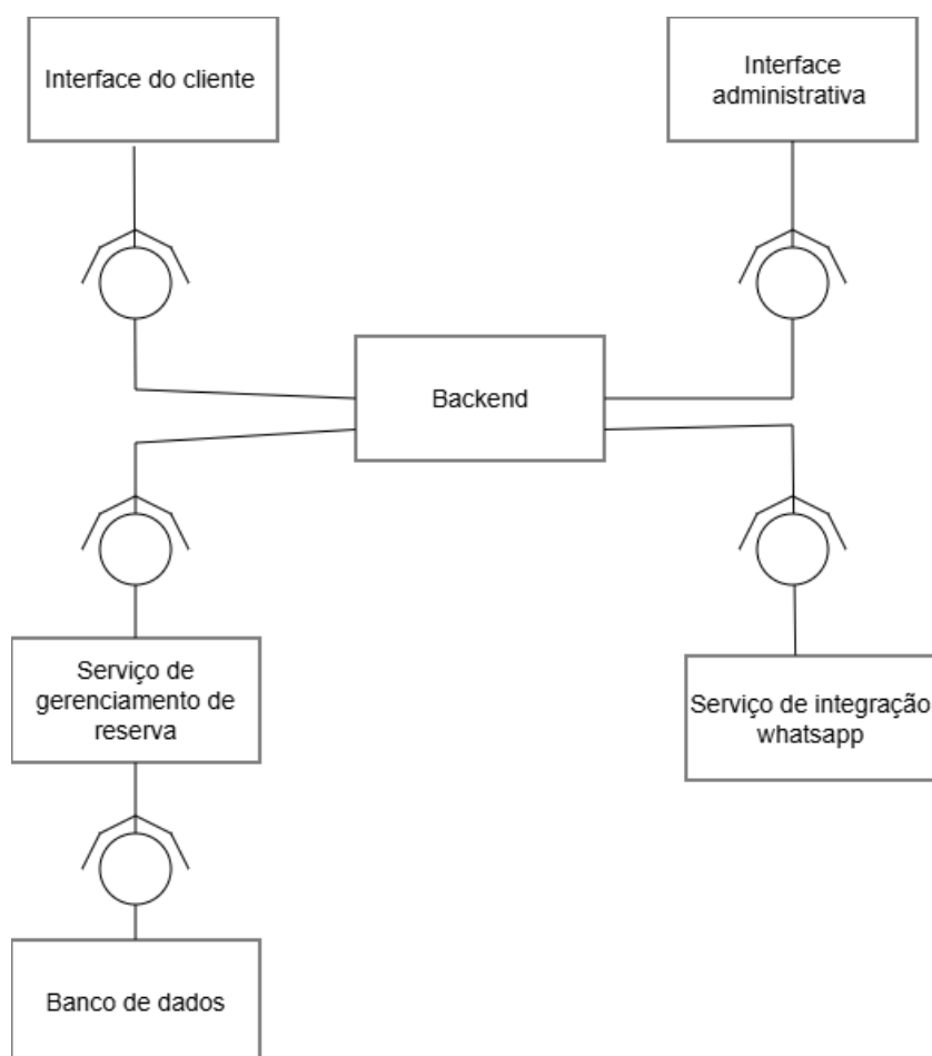
Imagem 08 – Diagrama de componentes
