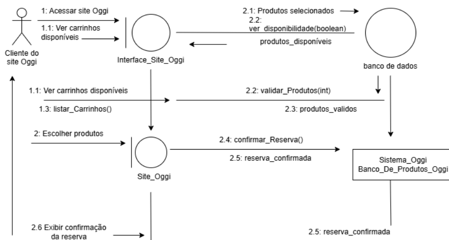
Imagem 05 – Diagrama de colaboração
