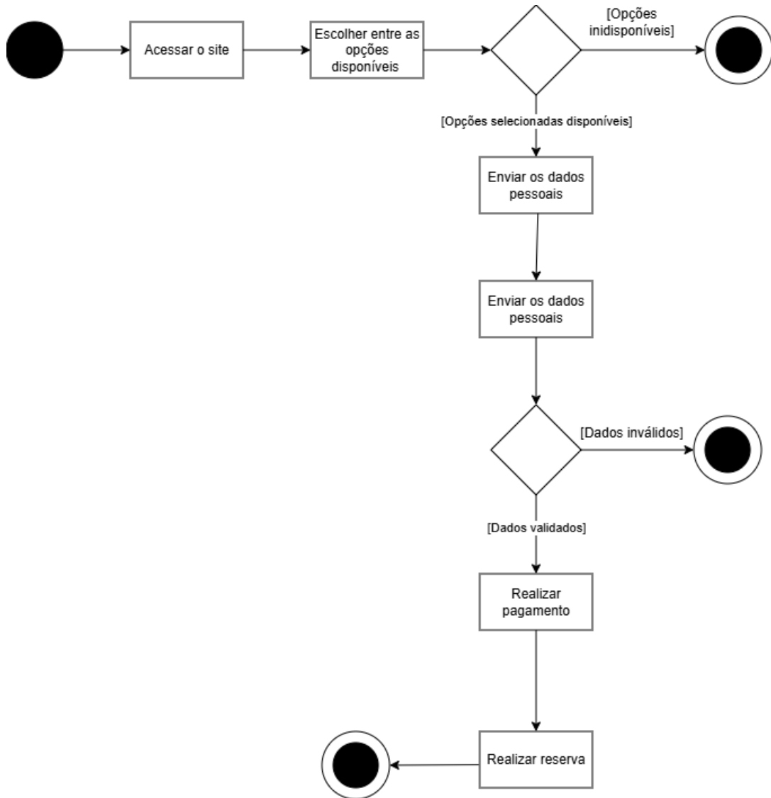
Imagem 07 – Diagrama de atividades
