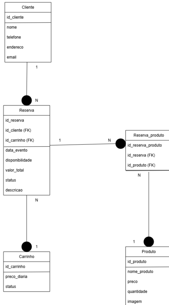
Imagem 11 – Modelo lógico
