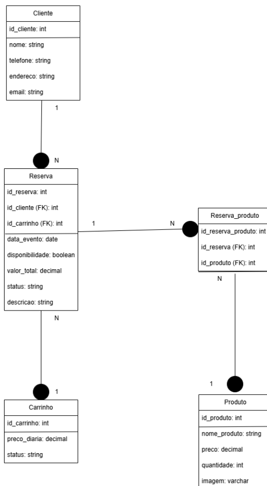
Imagem 12 – Modelo físico
