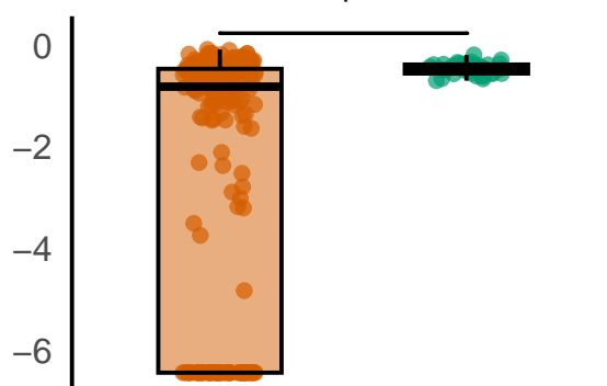
Lachnospiraceae
