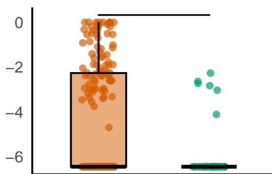
Enterococcaceae
