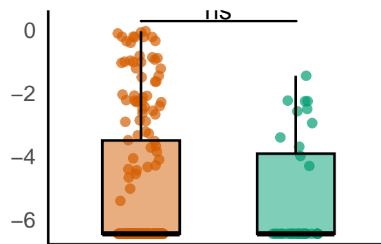
Enterobacteriaceae
