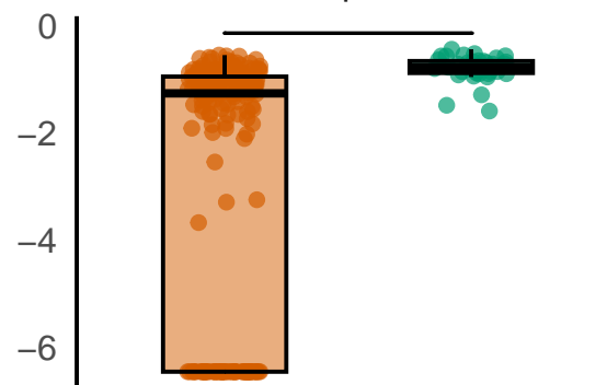
Oscillospiraceae
