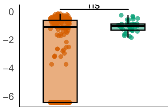
Bacteroidaceae
