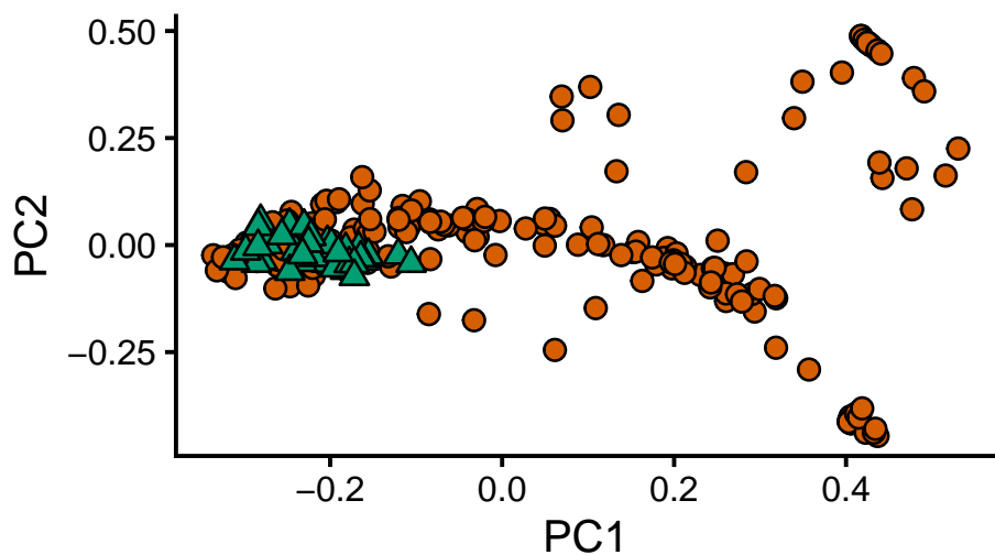
PCoA (Bray Curtis)
