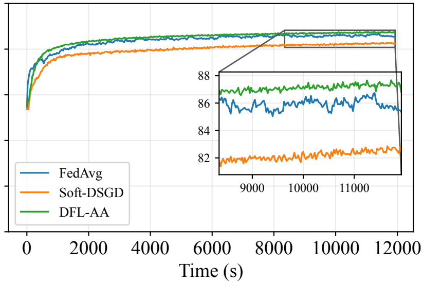
FMNIST (Dirichlet: 0.5)
