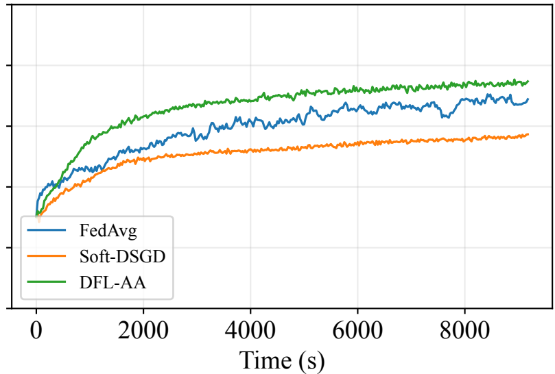
FMNIST (Dirichlet: 0.1)
