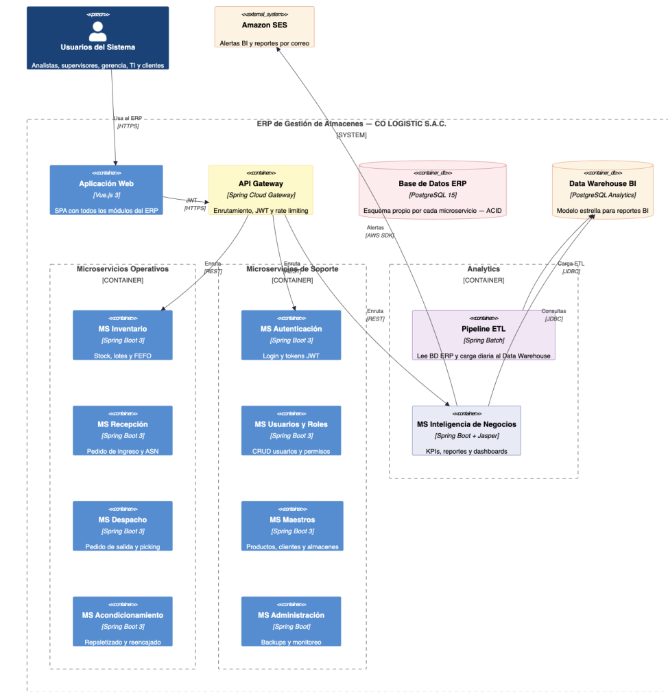
Figura 47. Arquitectura de microservicios de soporte al proceso automatizado
