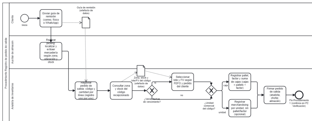
Figura 9. Diagrama BPMN — Registro de pedido de salida
