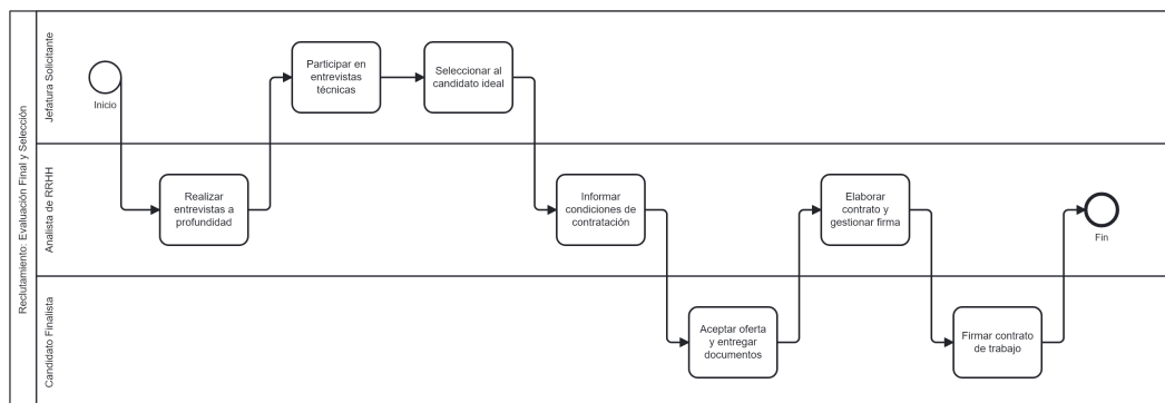
Figura 30. Diagrama BPMN — Evaluación final y selección
