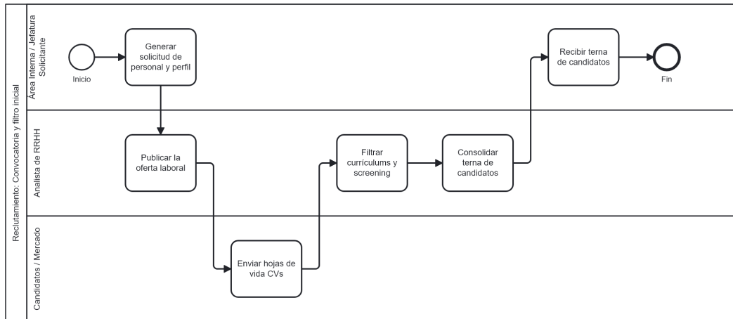
Figura 29. Diagrama BPMN — Convocatoria y filtro inicial
