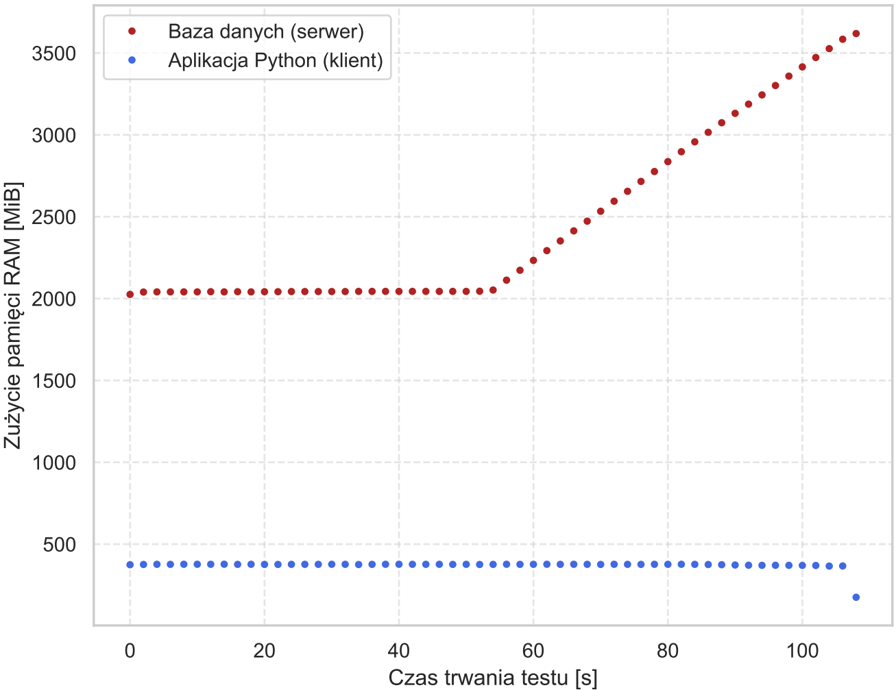
Zużycie pamięci RAM w czasie
