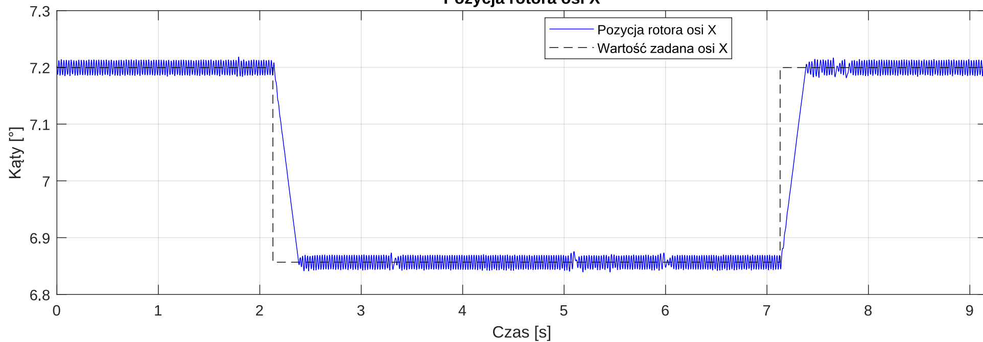
Pozycja rotora osi X
