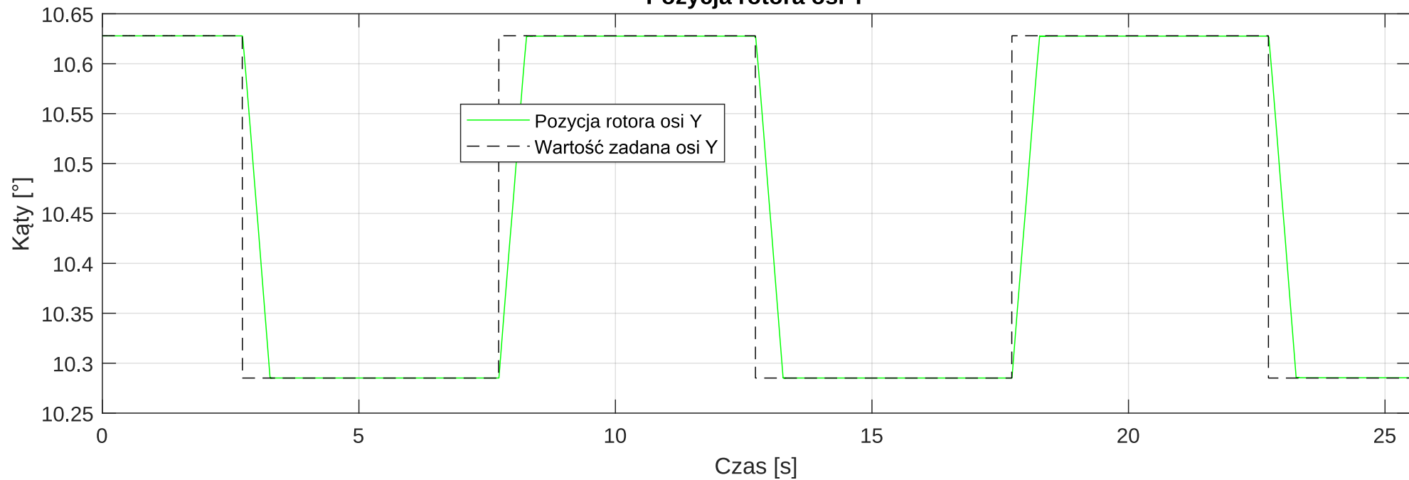
Pozycja rotora osi Y
