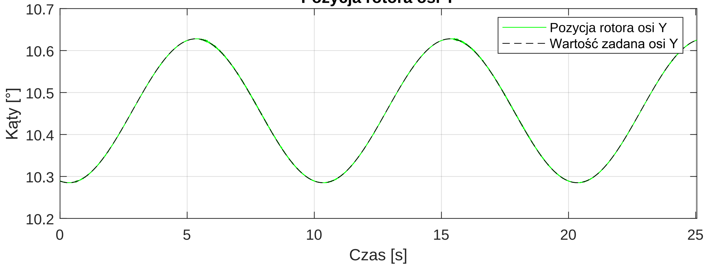
Pozycja rotora osi Y
